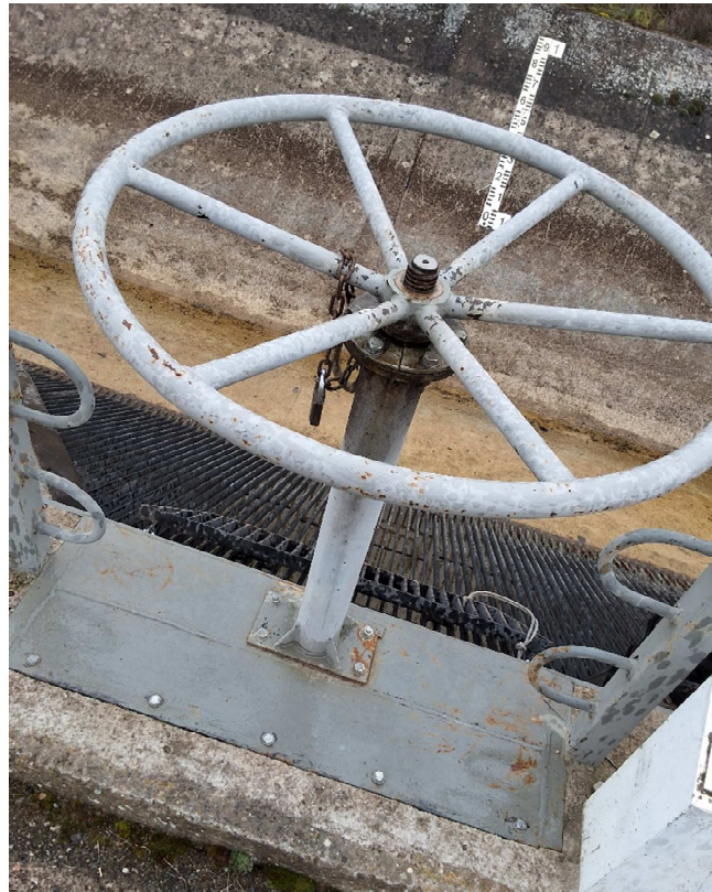
Fotografía 28 Compuerta S-9,520 en la Acequia de Selgua. Reja de desbaste.
